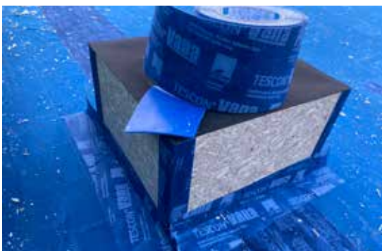
Zur sicheren Abdichtung von Durchdringungen
